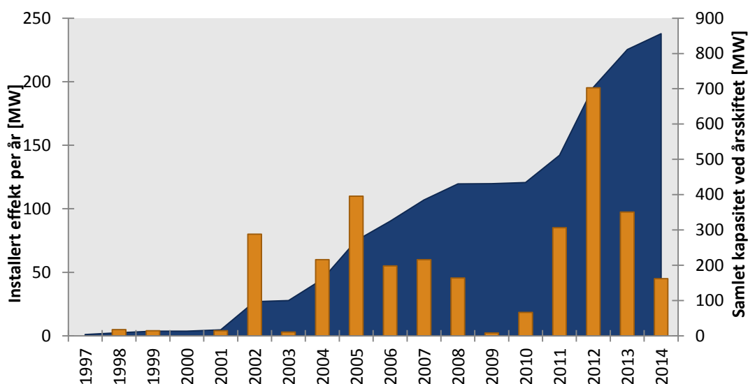
Figur 1 Installert vindkraft i Norge. Søylene og aksene til venstre viser installert effekt per år. Aksene til høyre og grafen viser samlet installert effekt ved årsskiftet hvert år.
