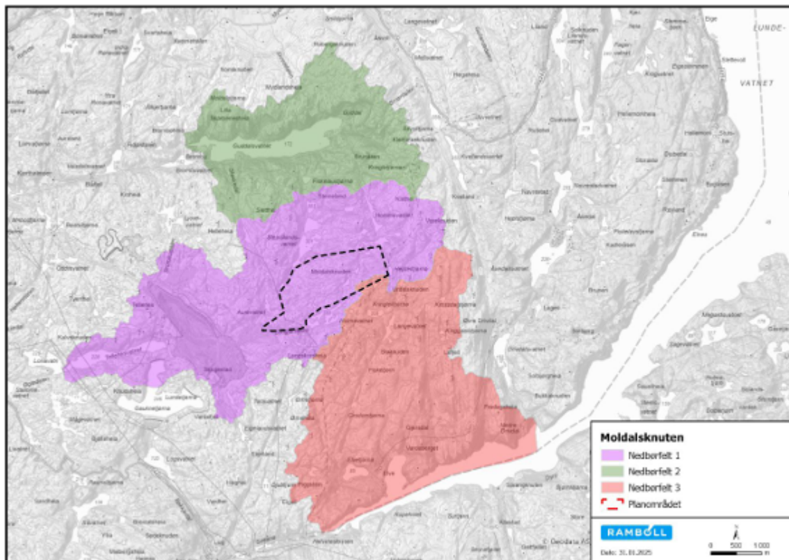
Figur 12 Oversikt over nedbørsfelt. Kilde: konsesjonssøknaden
