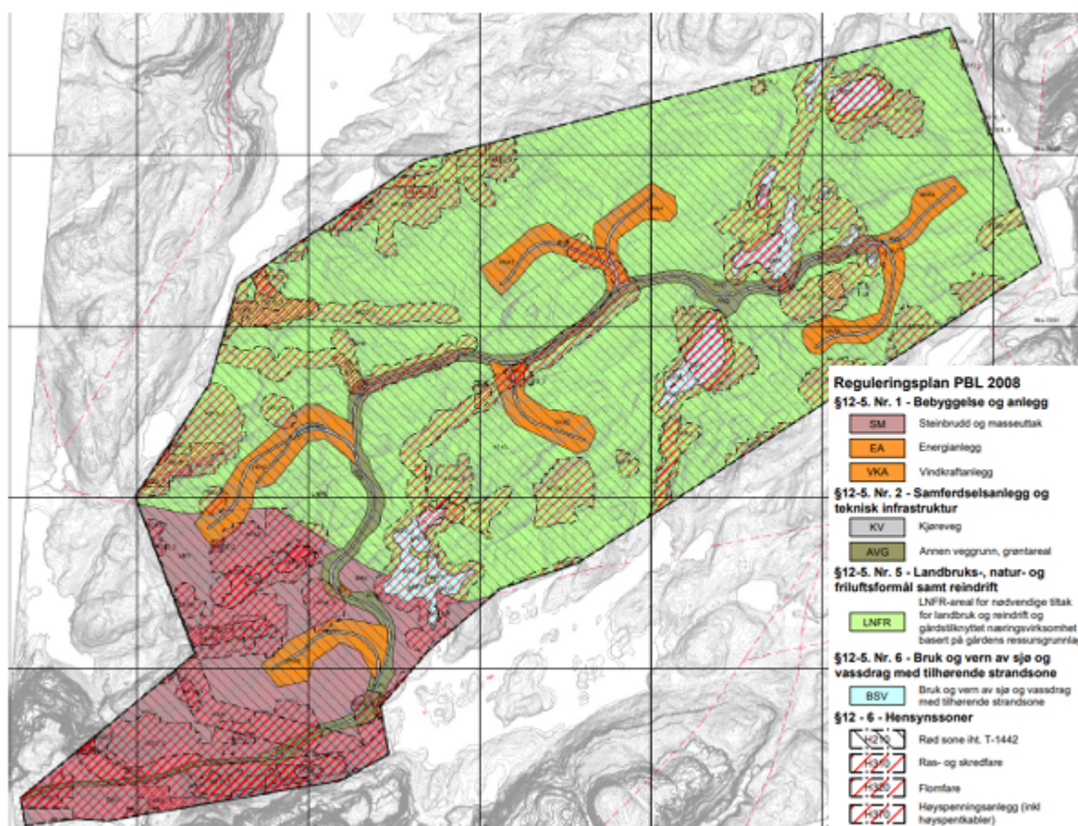
Figur 3 Plankart for Moldalsknuten vindkraftverk. Kilde: konsesjonssøknaden
