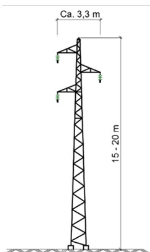
Figur 6 - Planlagt mast for luftledningen. Kilde: konsesjonssøknaden
