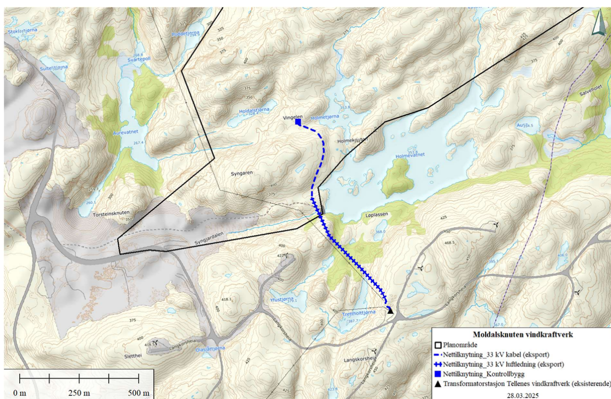
Figur 5 - Nettilknytning for Moldalsknuten vindkraftverk. Kilde: konsesjonssøknaden
