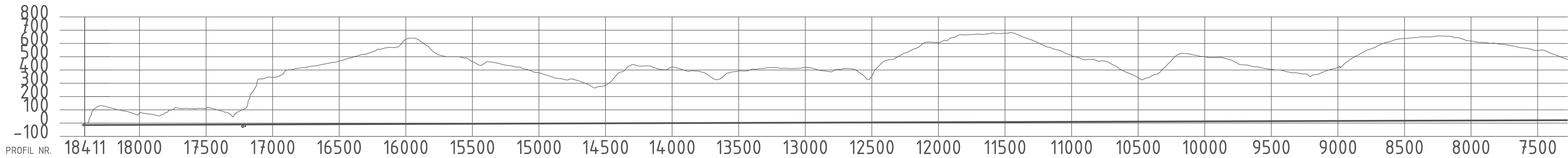
PROFIL: Tunnel Tiltak 5
