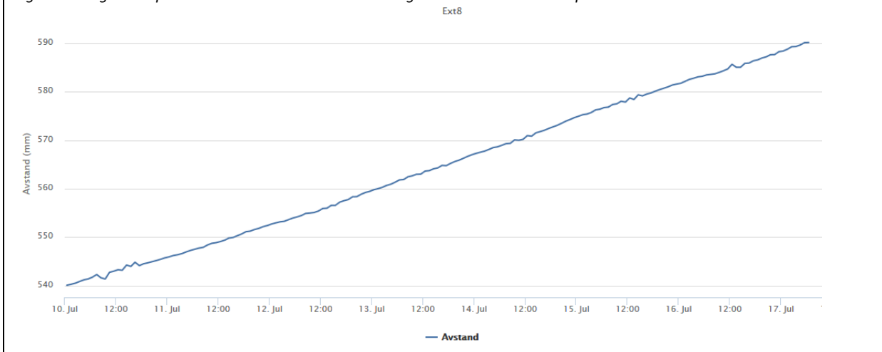
Figur 2 Bevegelsene på ekstensometer 8 den siste uka. Figur 1 viser hvor dette er plassert.
