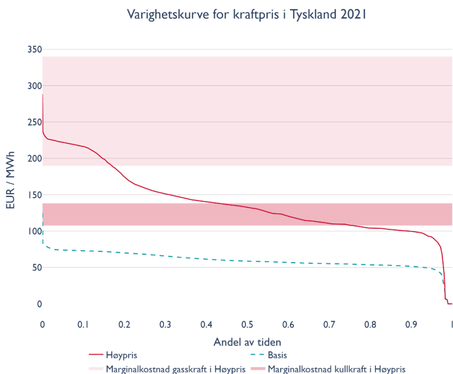
Figur 5: Varighetskurve med timespriser (øre/kWh) i alle værår for basis- og høyprisscenariet, samt utfallsrom for laveste og høyeste marginalkostnader til kull og gass i høyprisscenariet i Tyskland i 2021. Gjennomsnittlig kraftpris i Basis er 60 og i Høypris 139 €/MWh i Tyskland i 2021
