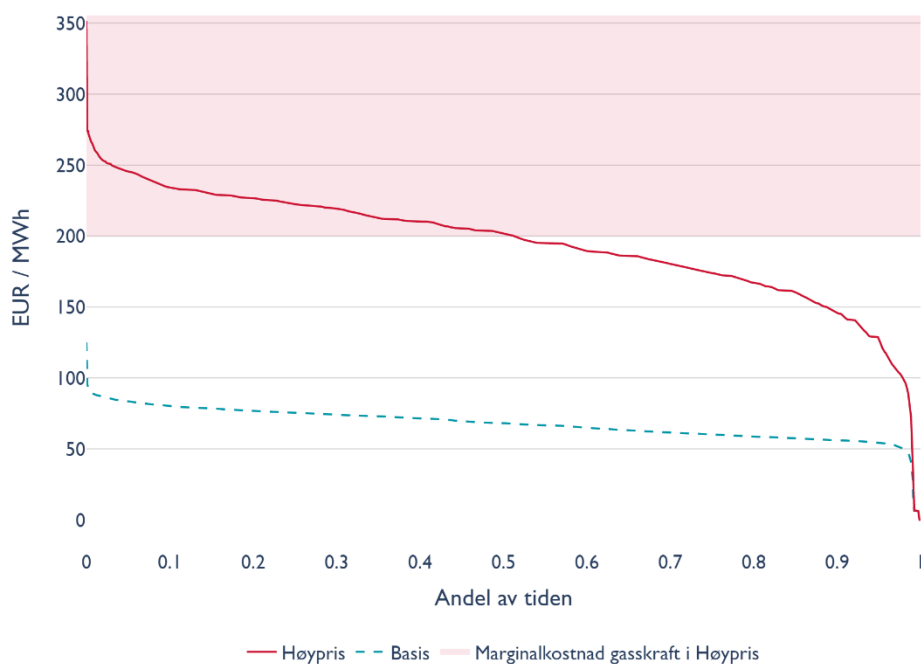
Figur 6. Varighetskurve med timespriser (øre/kWh) i alle værår for basis- og høyprisscenarioet, samt utfallsrom for lavest og høyeste marginalkostnader til kull og gass i høyprisscenariet i UK i 2021. Gjennomsnittlig kraftpris i Basis er 68 og i Høypris 195 €/MWh.
